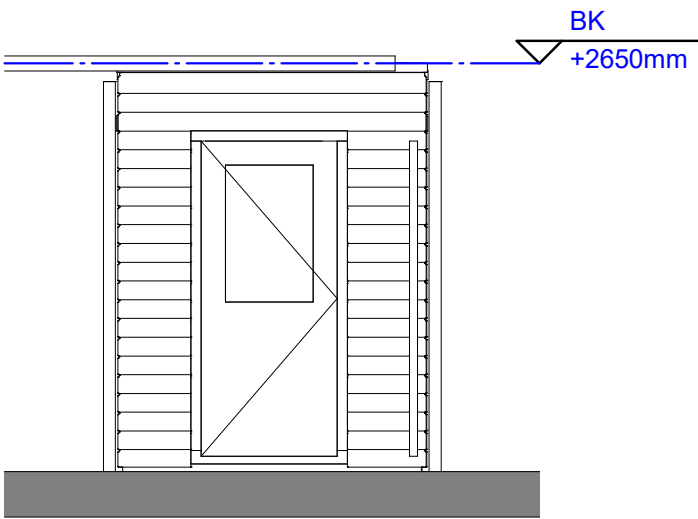
Linker zijaanzicht 1 : 50
