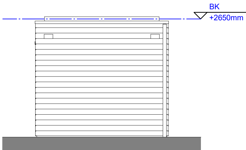
Achteraanzicht
