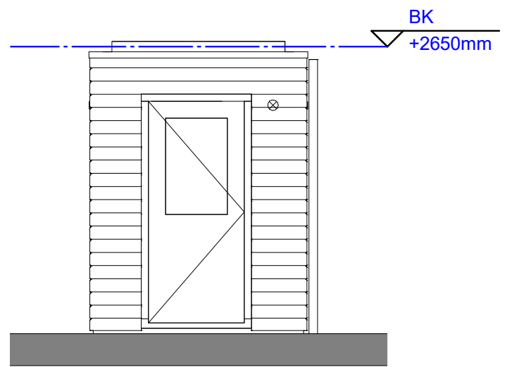
Rechter zijaanzicht
