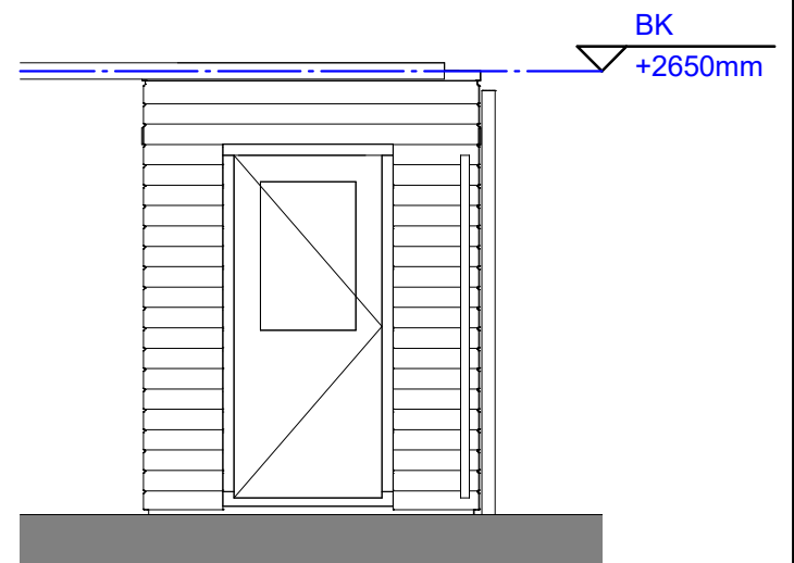
Linker zijaanzicht
