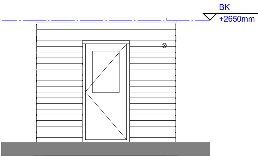
Rechter zijaanzicht 1 : 50
