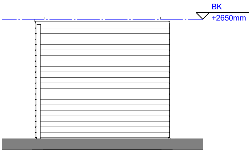
Linker zijaanzicht 1 : 50
