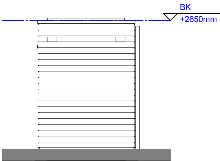
Achteraanzicht 1 : 50
