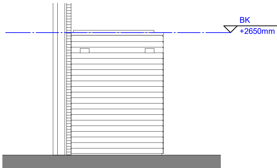
Vooraanzicht
