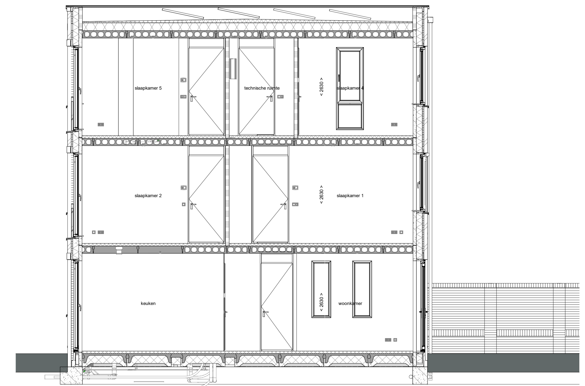
doorsnede A-A 1 : 50
