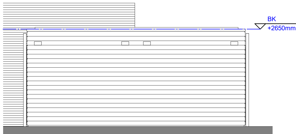
Vooraanzicht
