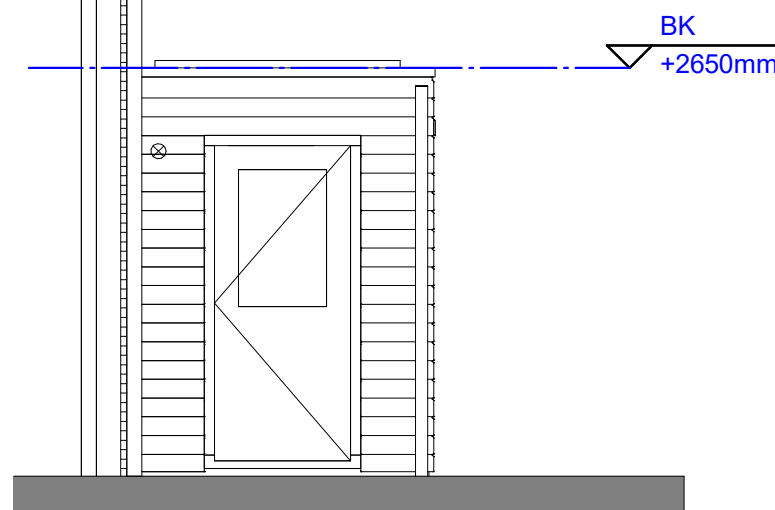
Rechter zijaanzicht
