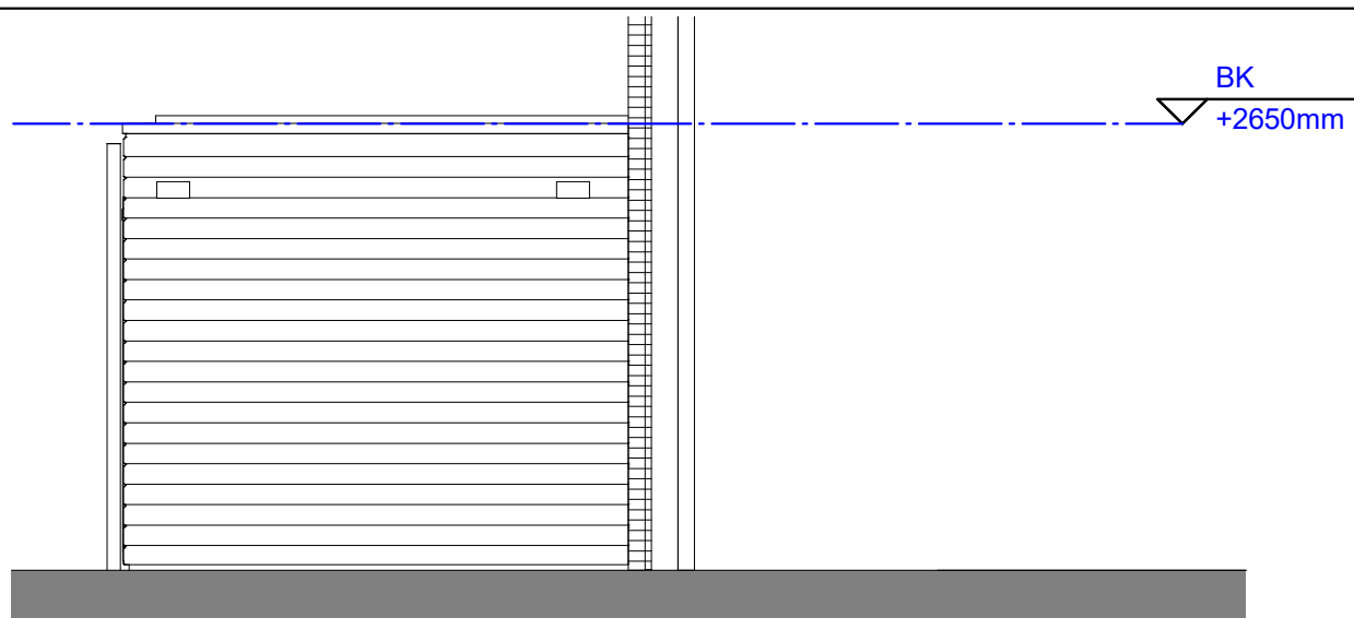
Vooraanzicht
