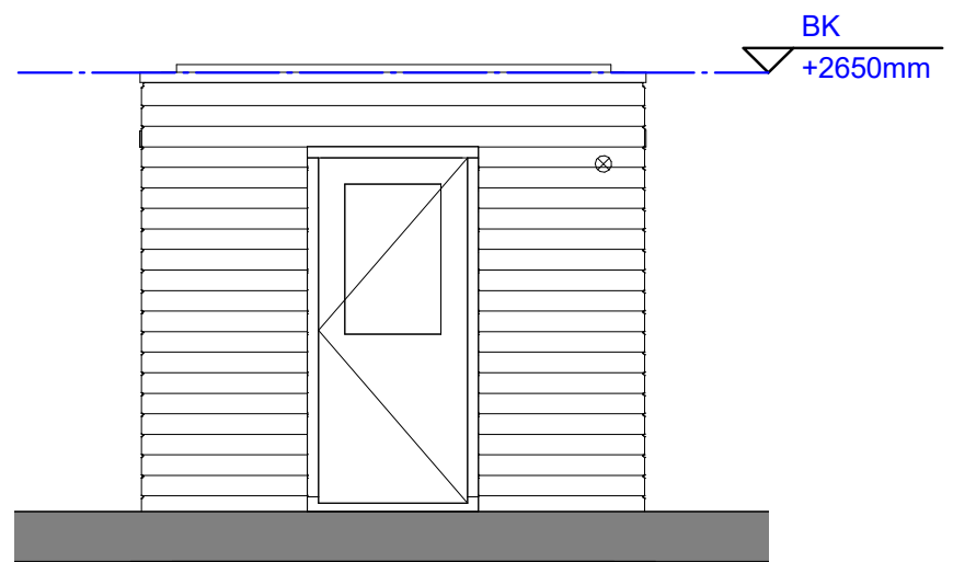
Rechter zijaanzicht
