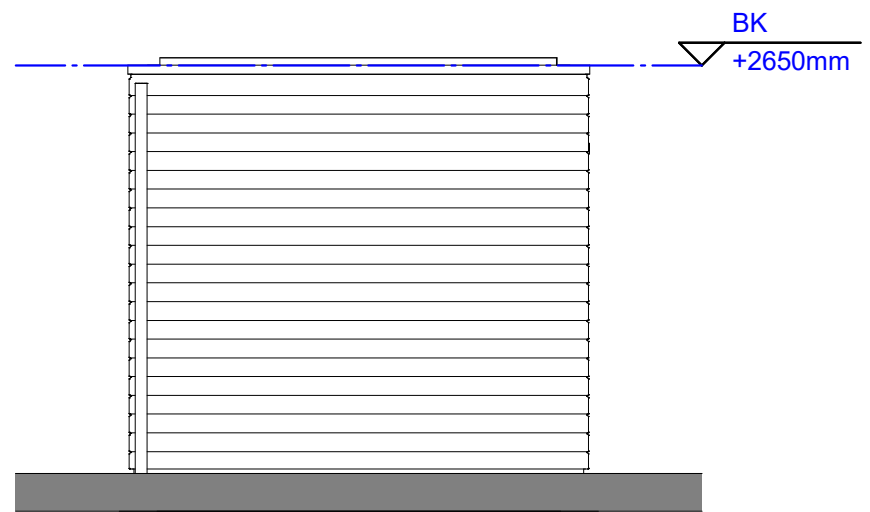
Linker zijaanzicht
